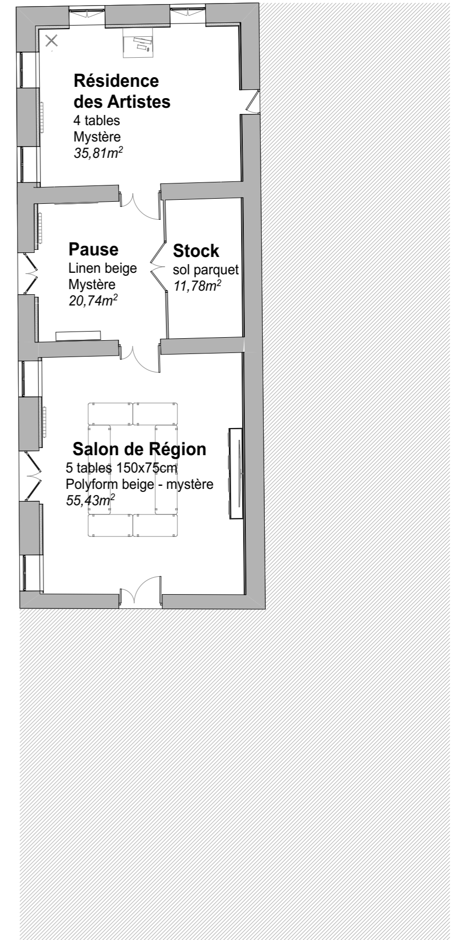
Plan du rez-de-jardin
